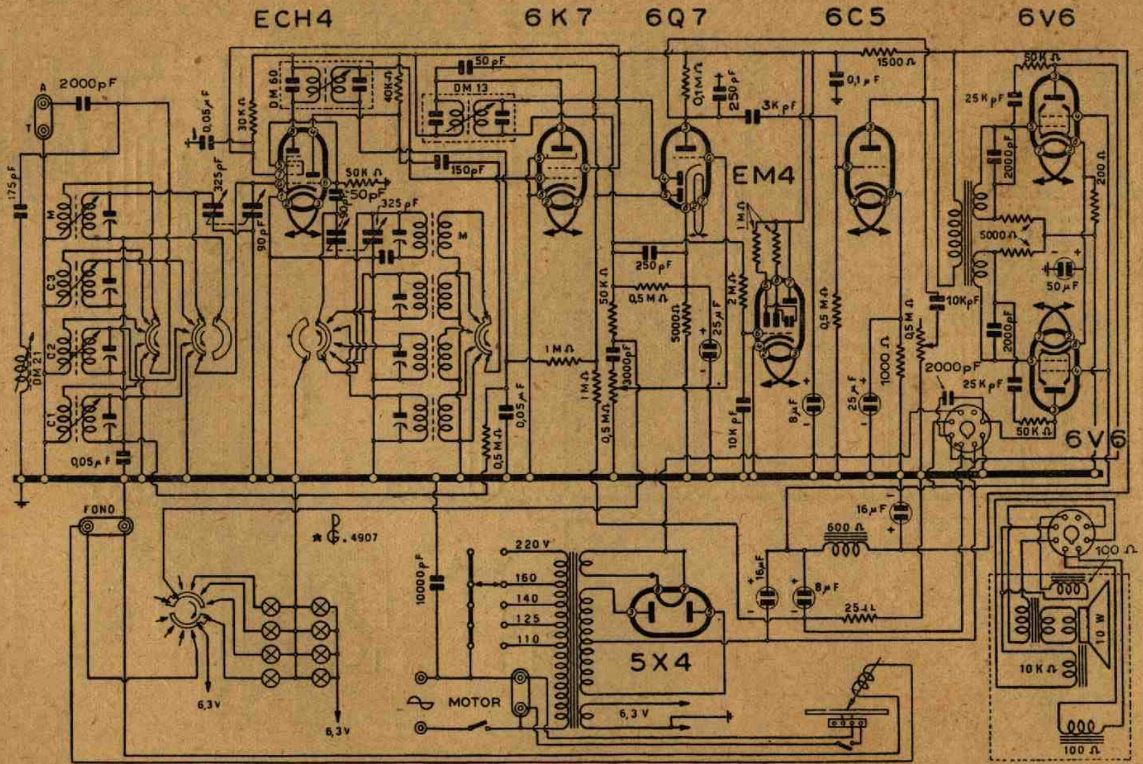
Lo schema elettrico del radiofonografo mod. 745 R F
